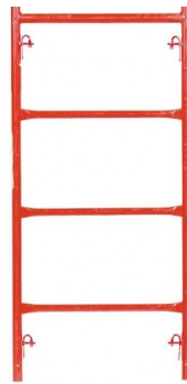
29” X 6'7” Ladder Frame
