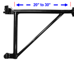
Adj. Side Bracket w/ Socket (tubular) "M" Hanger"
